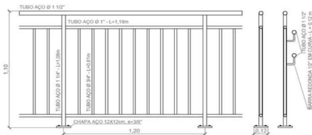
Detalhe do guarda-corpo
