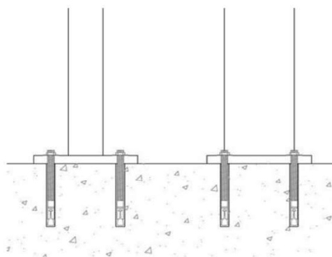
Detalhe da fixação do guarda-corpo
