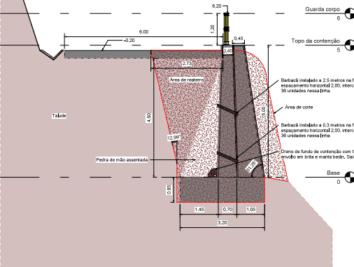
1 Corte esquemático 1 : 50
