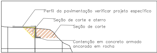
SEÇÃO TIPO ESCALA 1/200
