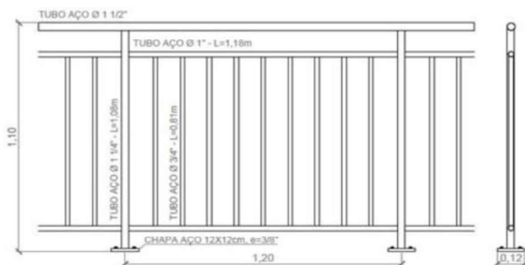
Croqui esquemático para confecção do guarda-corpo
