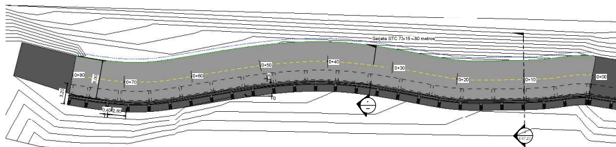
① Planta Baixa Contenção 1 : 200
