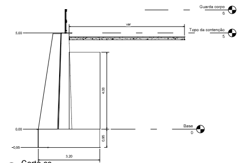
② Corte cc 1 : 50
