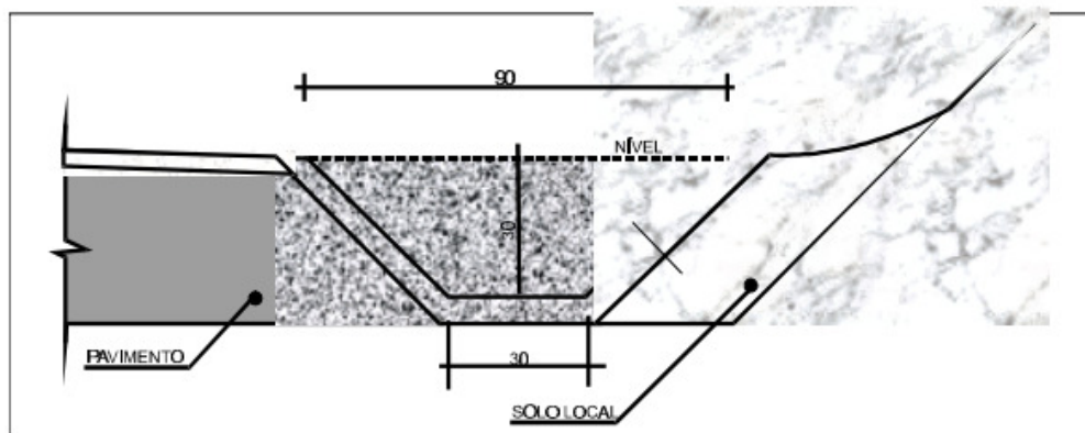
Figura 03. Sarjeta Trapezoidal de Concreto Tipo SZC01
