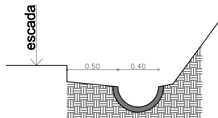
VALETA DE CONCRETO ( lado oposto barranco/corrimão)
