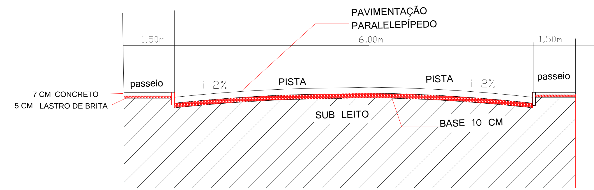
SEÇÃO -TIPO 1
