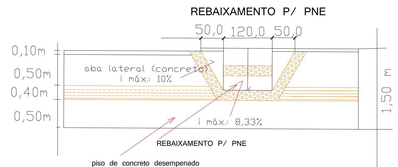
DETALHAMENTO DO PISO TATIL DO PASSEIO
