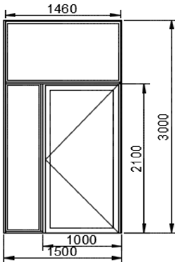
FIG : 1 porta de giro - 1 caixilho lateral fixo - 1 bandeira fixa
