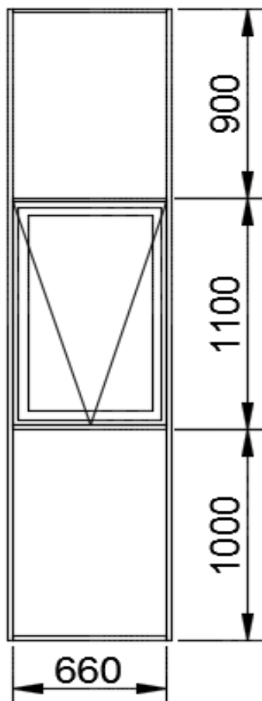
Fig : 1 peitoril fixo - 1 janela maxiar - 1 bandeira fixa
