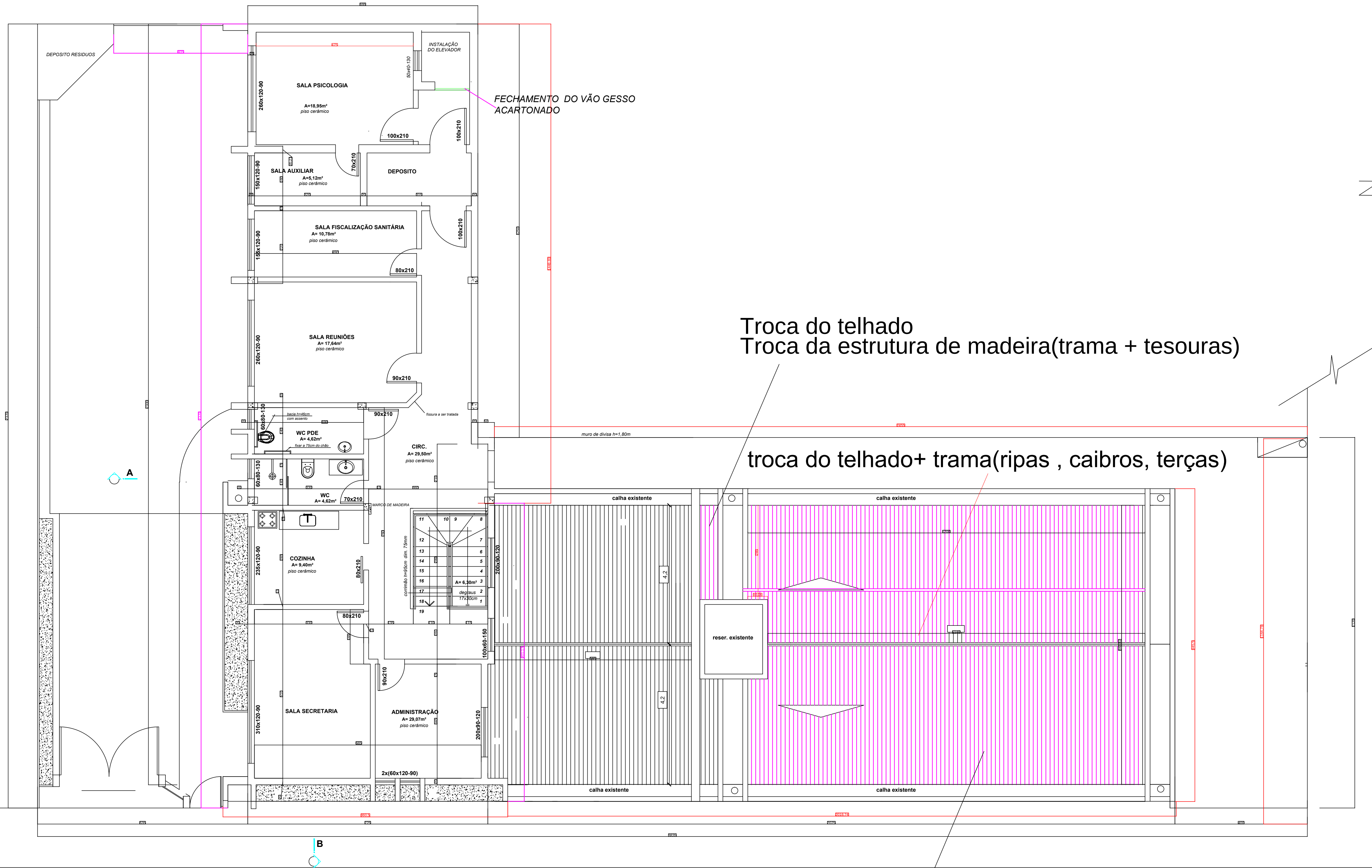
PLANTA BAIXA - Pav. Superior A=168,48m2 A total= 292,28m2 Esc.: 1/75
