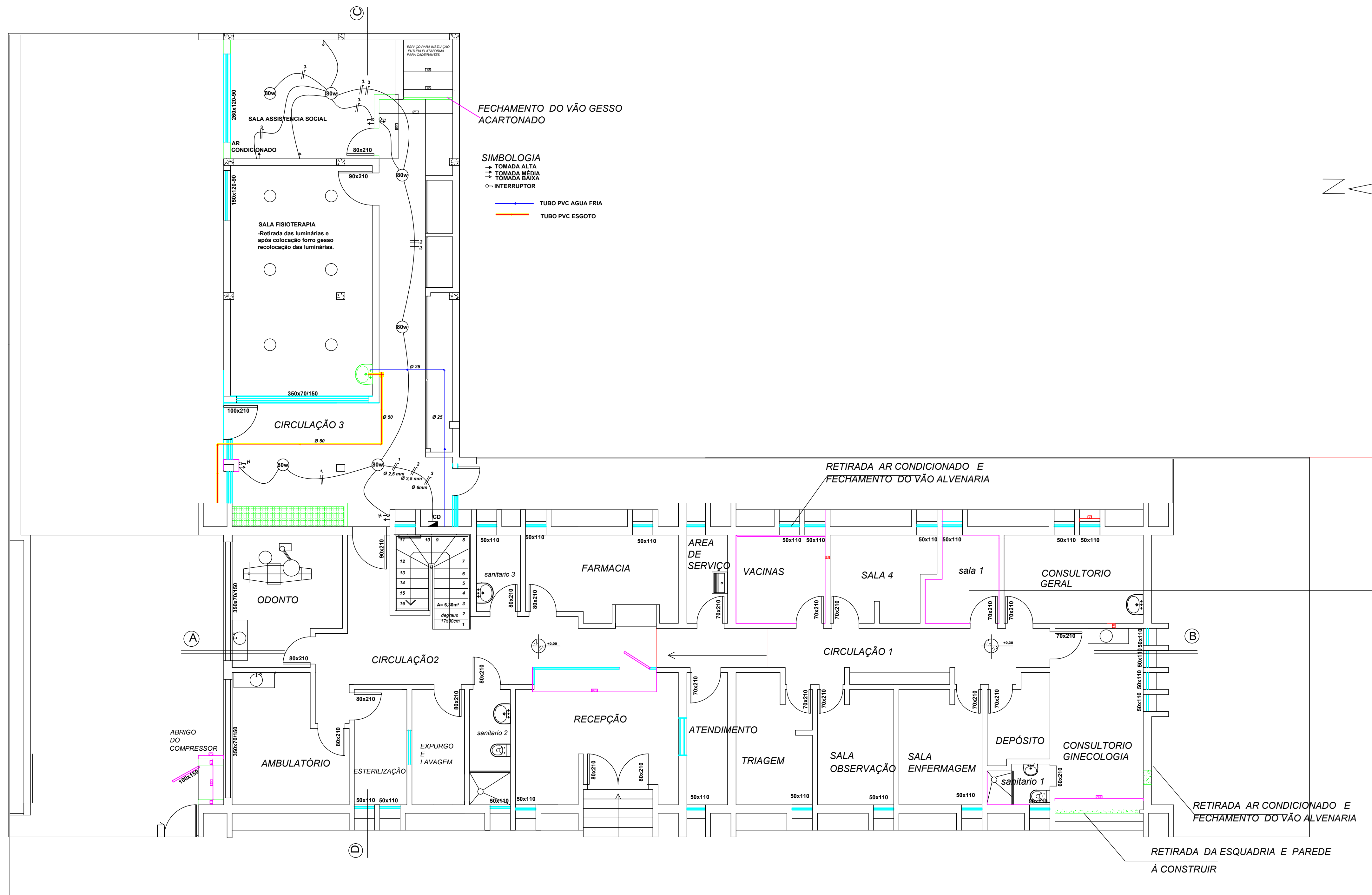
PLANTA BAIXA
