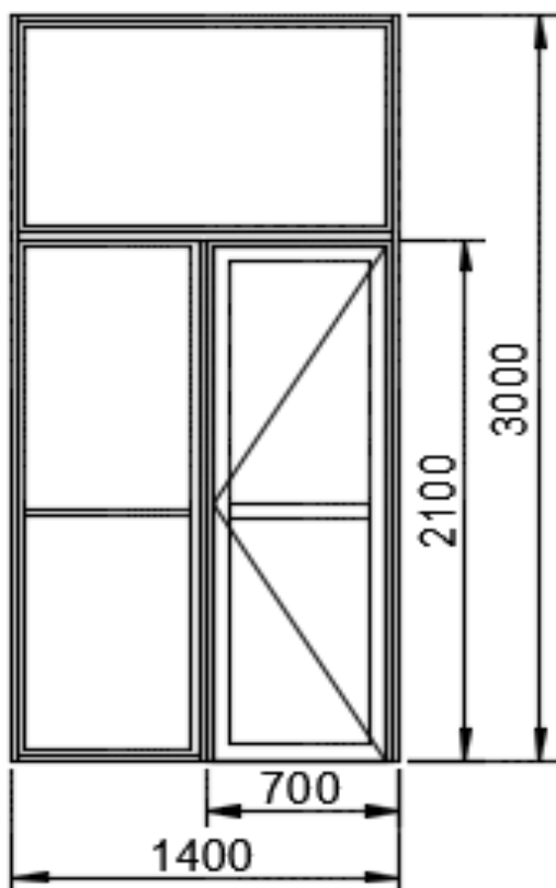
Fig: 1 porta de giro - 1 caixilho lateral fixo - 1 bandeira fixa
