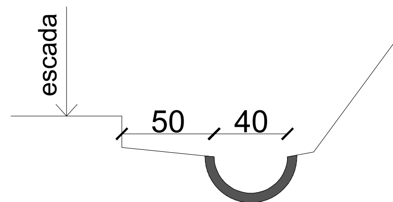
VALETA DE CONCRETO (lado oposto ao barranco)
