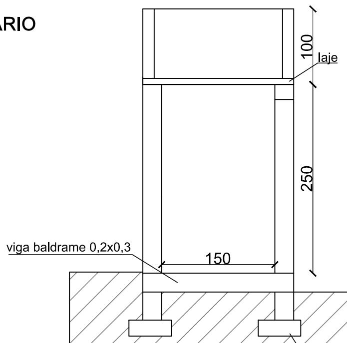
CORTE TRANSVERSAL 1 | 50
