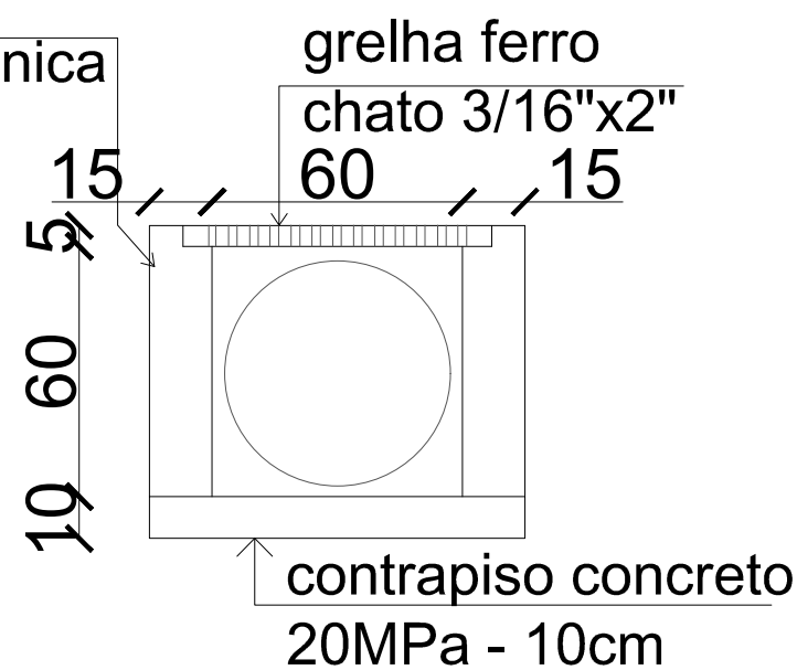
corte esquemático CAIXA DE PASSAGEM *a cada 25m aprox.
