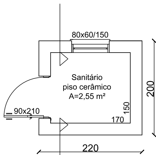
PLANTA BAIXA SANITÁRIO 1 | 50
