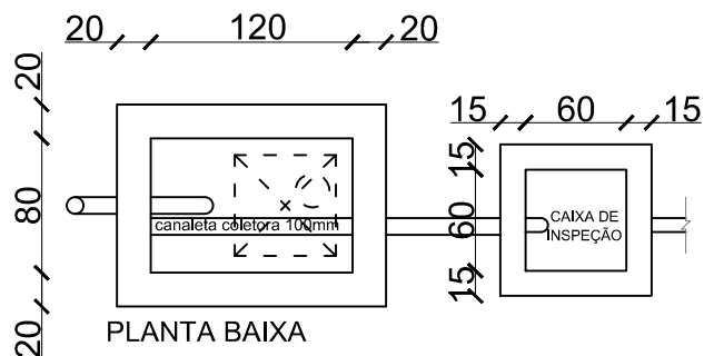
FILTRO ANAERÓBIO Volume: 1152 L Para: 5 contribuintes
