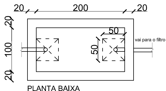
TANQUE SÉPTICO Volume: 2000 L Para: 5 contribuintes
