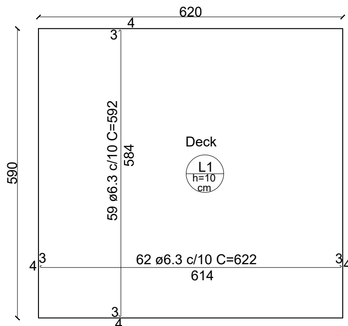
Laje - Armadura Principal (Positiva) Escala: 1/75
