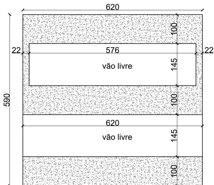
Planta Baixa Térreo - Estrutura de Concreto Existente
