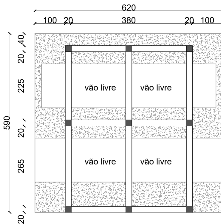
Planta Baixa Locação de Vigas e Pilares
