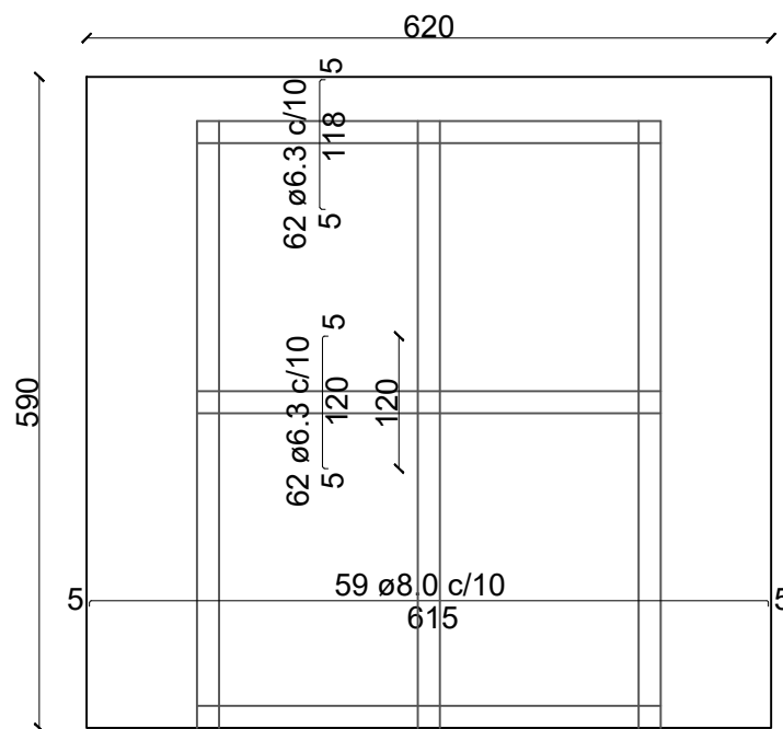
Laje - Armadura Negativa Escala: 1/75
