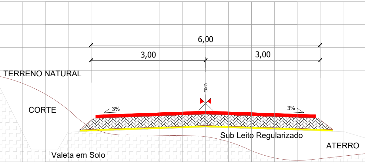
SEÇÃO TRANSVERSAL TIPO (EM TANGENTE)
