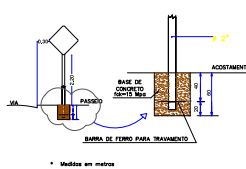
Detalhe Fixação Simples de Placas
