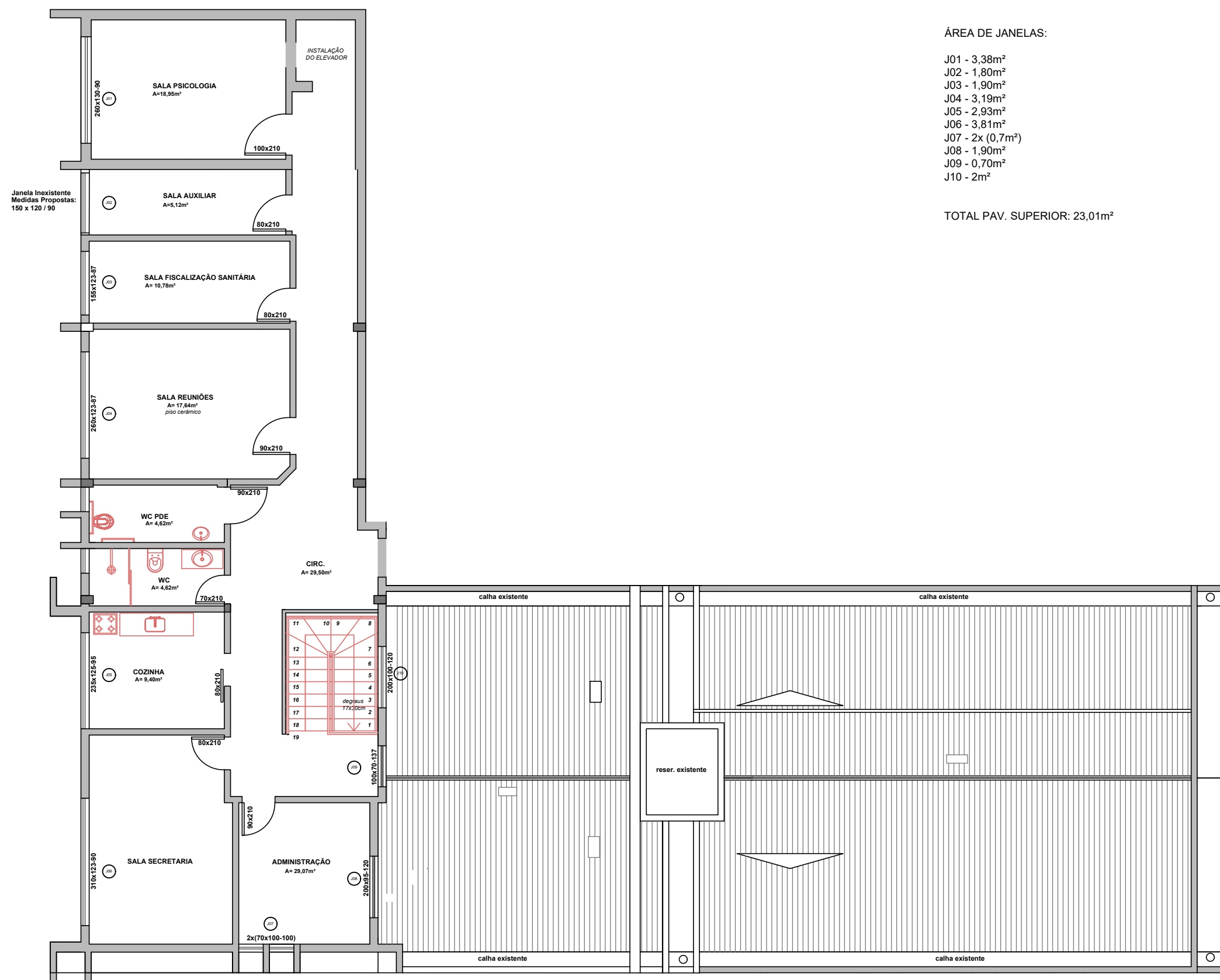
PLANTA BAIXA - Pav. Superior
